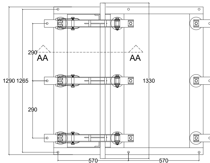
CORTE AA
